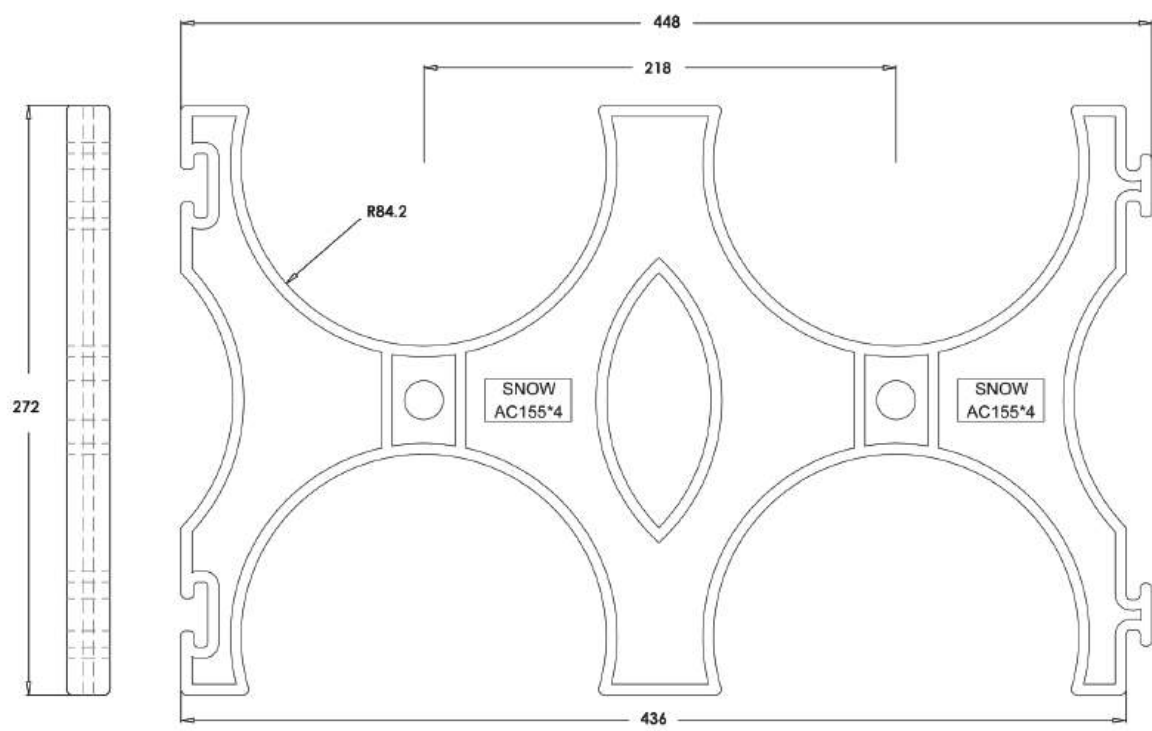
6''*2 Holes CL B Arches Spacer (P.P.)
