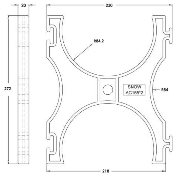
6''*2 Holes CL B Arches Spacer (P.P.)
